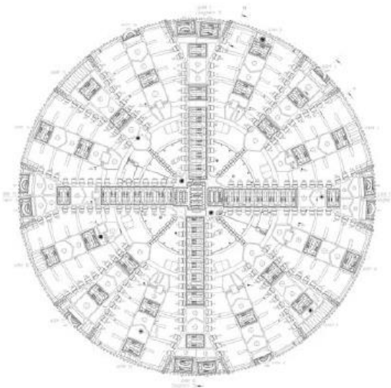
Nova roda de tall híbrida
