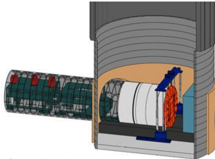
Grua auxiliar a l'interior del pou
