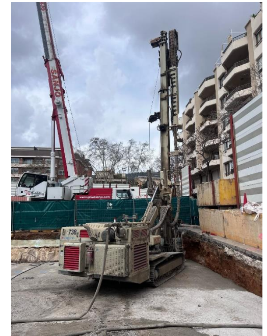
Execució fonamentació grues
