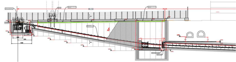
Secció tram pou arribada i trinxera a l'alçada de Llança
