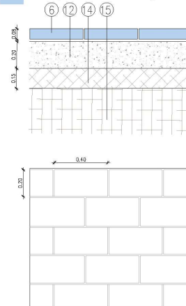
Llosa prefabricada formigó 60x40
