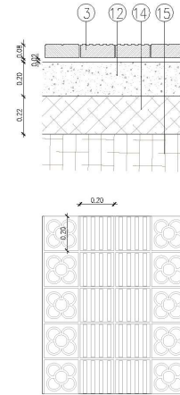
Lloseta prefabricada de morter. Panot amb botunadura (senyalització)
