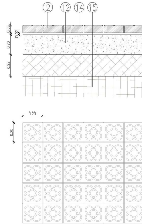
Lloseta prefabricada de morter. Panot 8cm Flor
