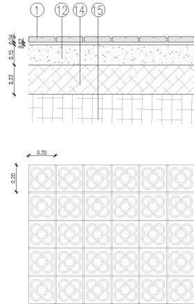
Lloseta prefabricada de morter. Panot 4cm Flor
