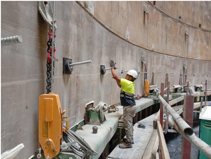
13. Col·locació capçals ancoratges actius anell anterior
