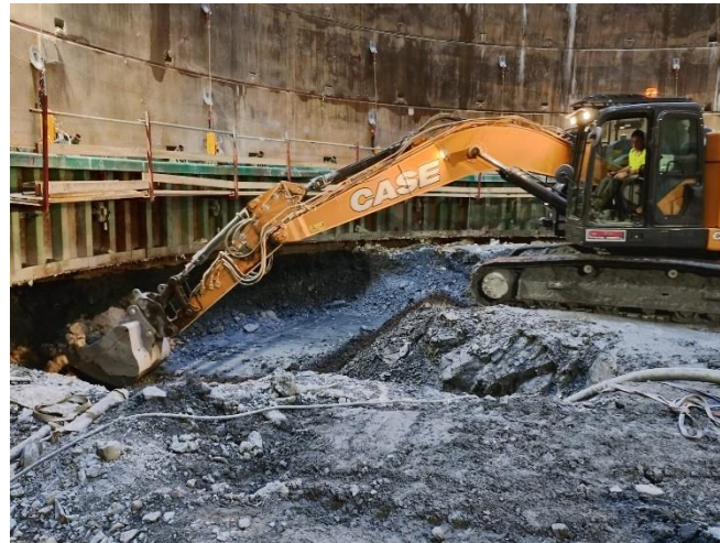
1. Demolició formigó de neteja i excavació anell
