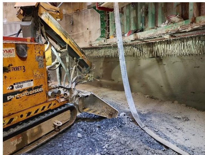
3. Gunitat trasdós anell
